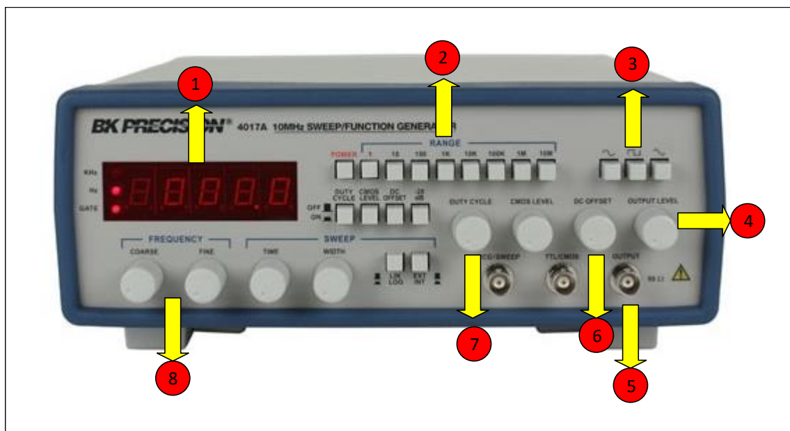
Figura 15. Generador de Señales
