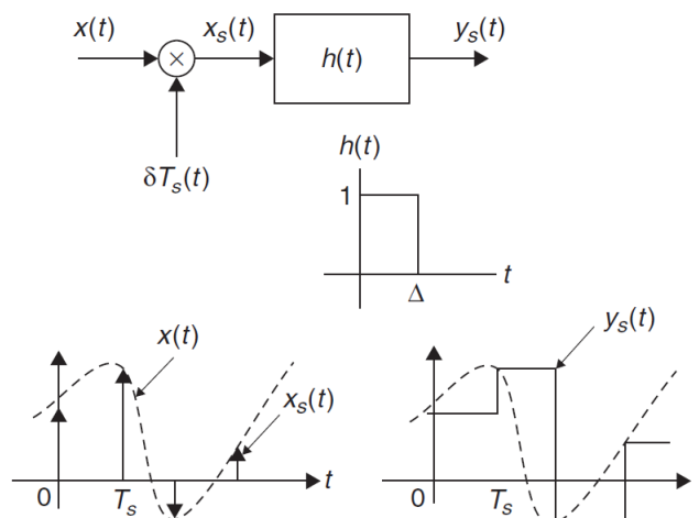
Figura 19. Muestro utilizando un sistema de muestreo y retención
