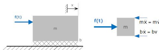
Figura 17. Acción de una fuerza sobre una masa.
