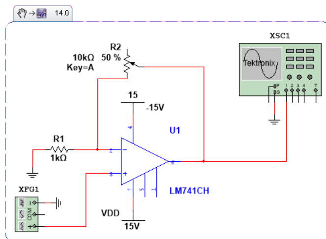
Figura 9. Circuito dos
