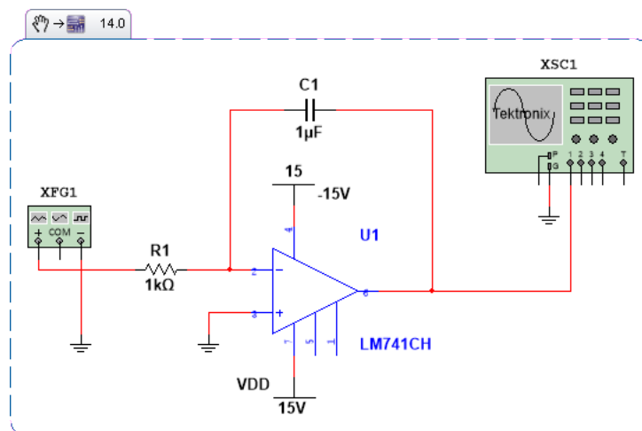
Figura 7. Circuito uno
