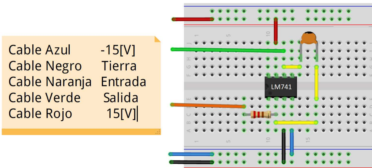
Figura 8. Circuito uno
