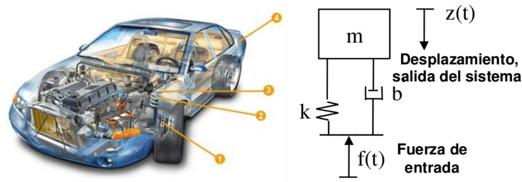
Figura 24. Modelo del sistema de suspensión
