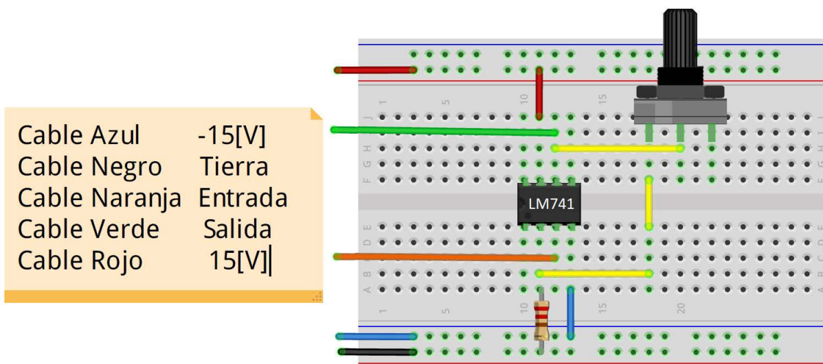
Figura 10. Circuito dos
